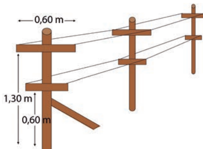
Figura 3. 1. Sistema de conducción tipo doble cruceta en frambuesa.
